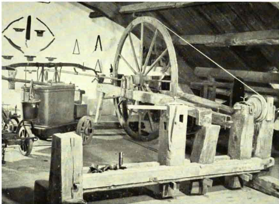
Draaibank (cat. 167)
